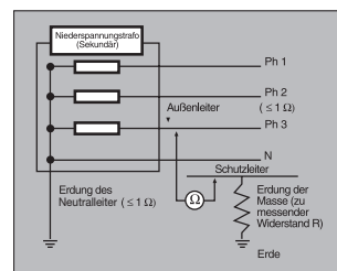
Prinzip der Schleifenwiderstandsmessung / Neutralleiter liegt auf Erde
