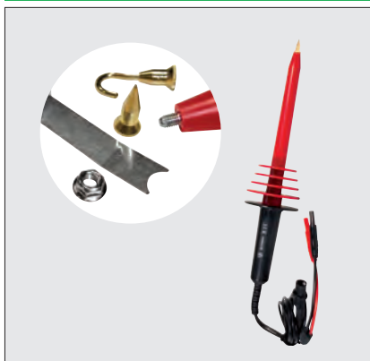
Hochspannungstastkopf SHT 40 kV für Multimeter P01102097 ■ Maximale zulässige Spannung: 40 kV DC , 28 kV eff bzw. 40 kV Spitze (50/60 Hz) ■ Wandlerverhältnis (Eingang / Ausgang): 1 kV/1 V ■ Für Multimeter mit Eingangsimpedanz von 10 MΩ
