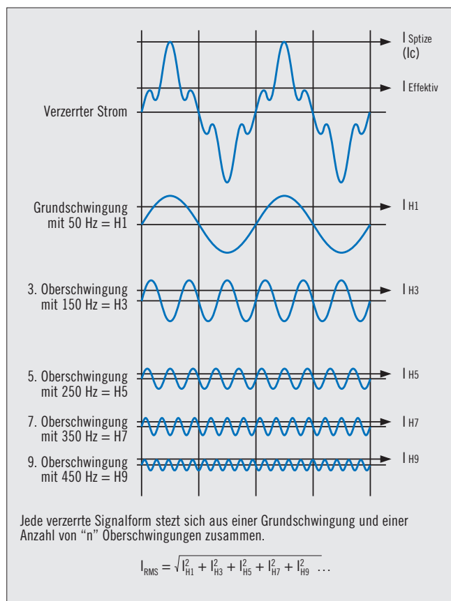
Abb. 1 - Beispiel eines verzerrten AC-Stroms mit ungeraden Oberschwingungen (3, 5, 7, 9, ...)
