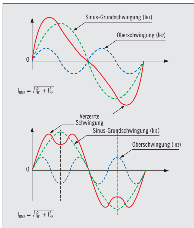
Abb. 2 - Zerlegung einer verzerrten Schwingung in Grundschwingung und Oberschwingung 2. bzw. 3. Ordnung
