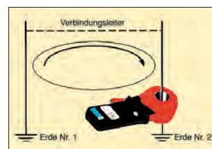
Prinzip der Basis-Schleife: sie besteht aus zwei lokalen Erdungen, die mit einem Leiter verbunden werden.
