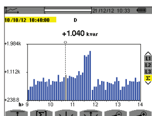
Darstellung des Lastprofils
