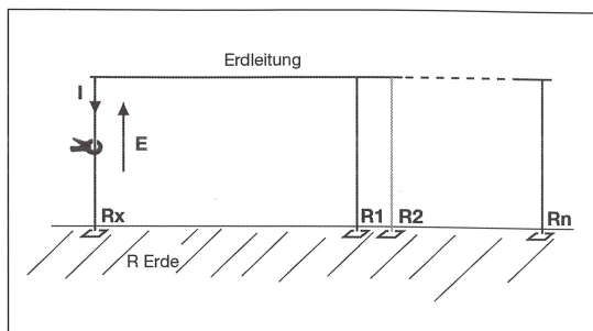
Schaltbild der Prüfung mit Erdungsprüfzange
